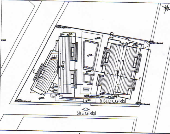
VAZİYET PLANI
